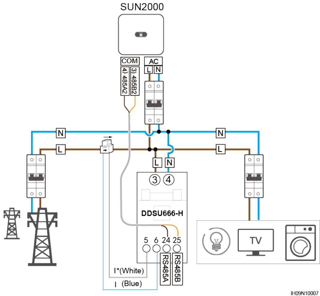
Figura 5-29 Conexión de los cables al contador de potencia DDSU666-H
