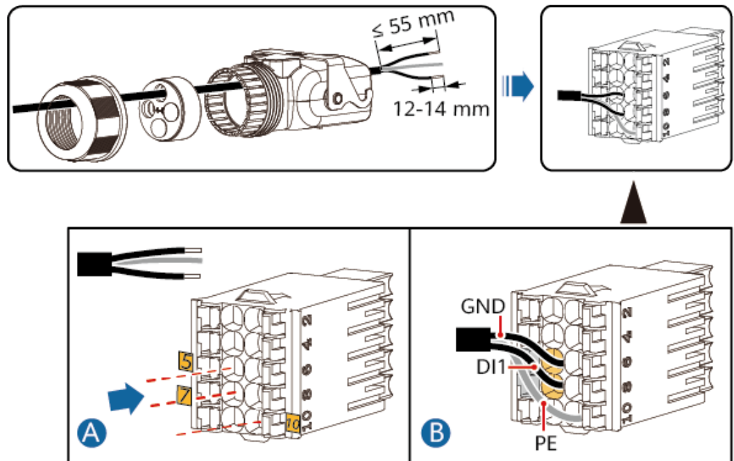
Figura 5-33 Instalación del cable
