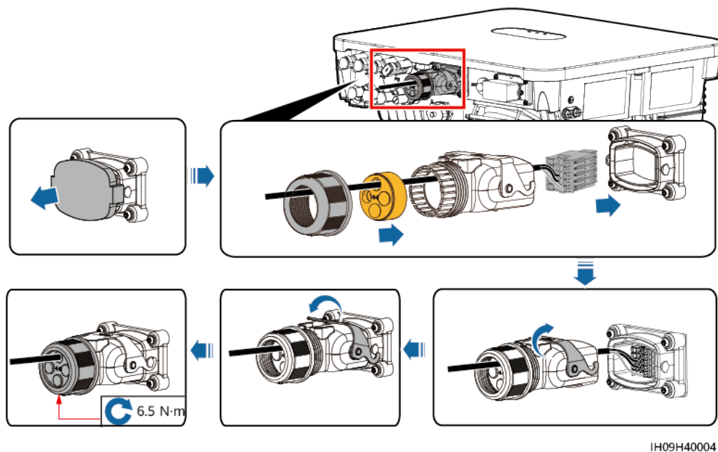
Figura 5-34 Fijación del conector del cable de señal
