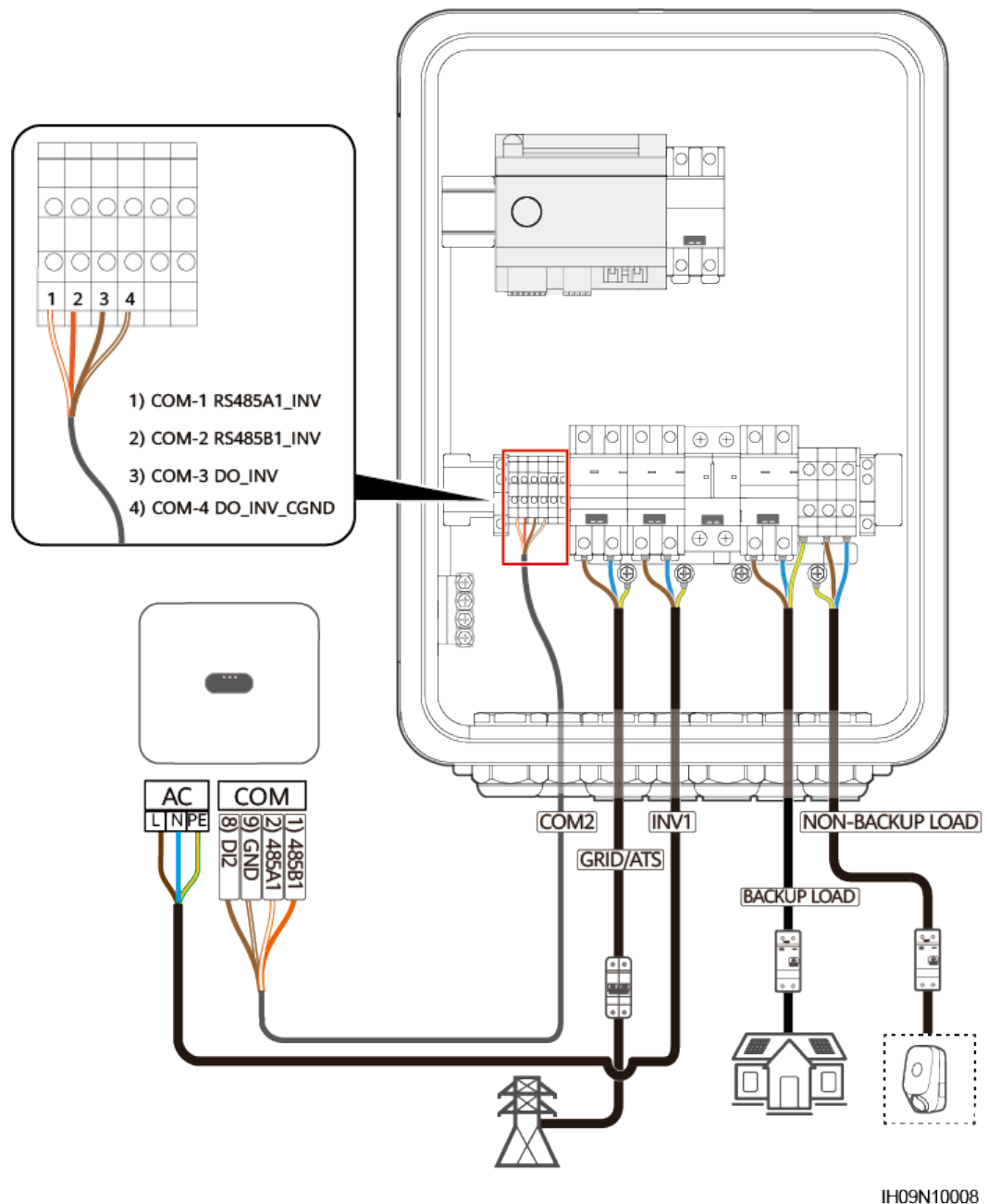
Figura 5-25 Conexión de los cables al SmartGuard
