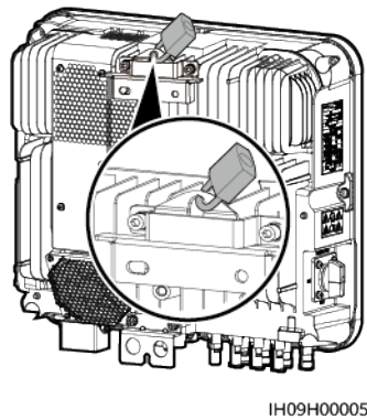
Figura 4-10 Instalación de un candado antirrobo
