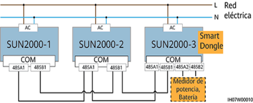
Figura 5-14 Conexión en red del Smart Dongle (los componentes opcionales están encerrados en un cuadro de rayas pequeñas)
