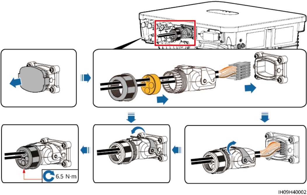
Figura 5-24 Fijación del conector del cable de señal
