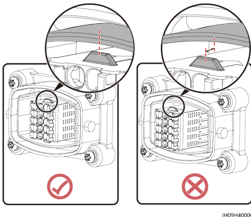
Figura 5-18 Instalación del bloque de conectores
