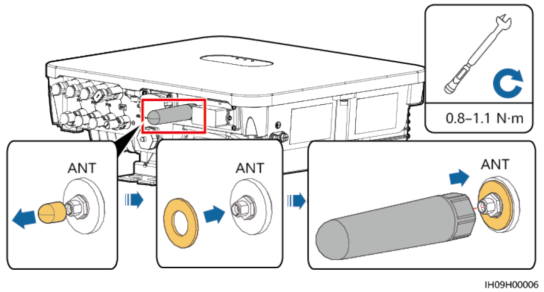
Figura 5-39 Instalación de una antena WLAN
