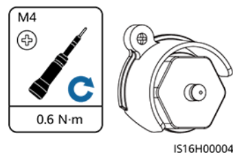
Figura 5-38 Instalación de componentes antirrobo para el Smart Dongle
