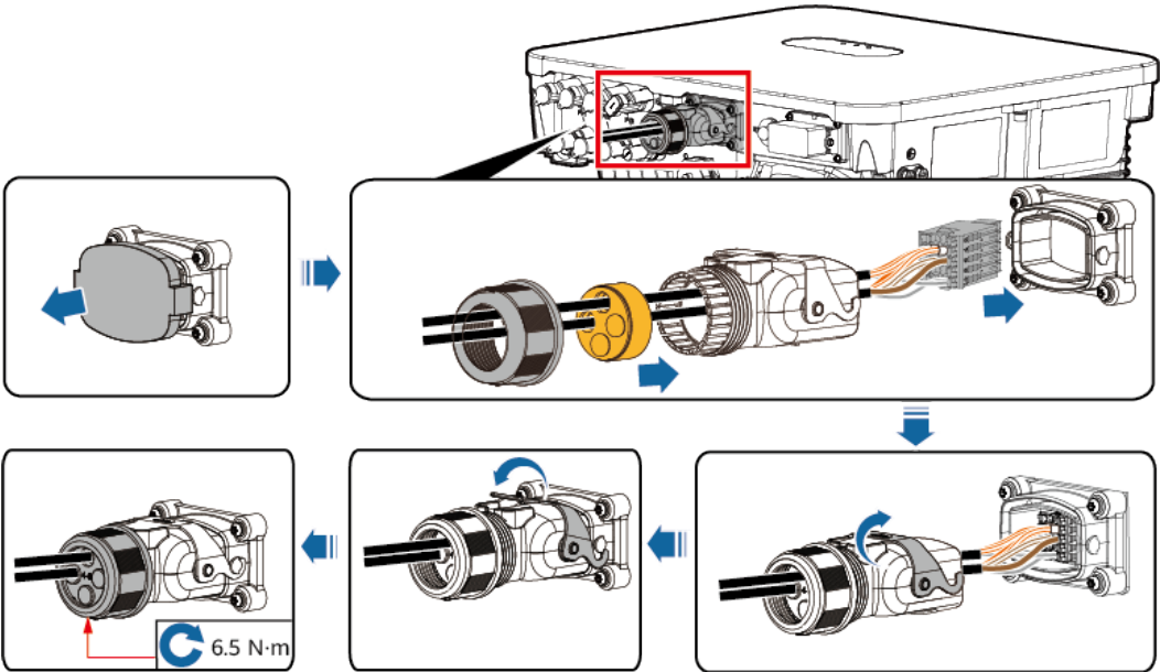
Figura 5-32 Fijación del conector del cable de señal
