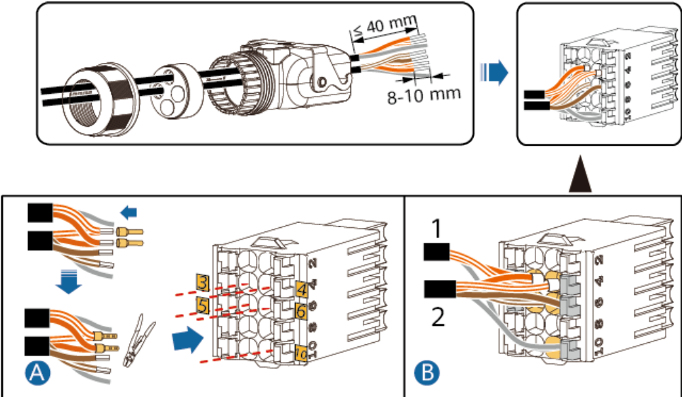
Figura 5-31 Instalación de los cables (conexión al contador de potencia y a la batería)
