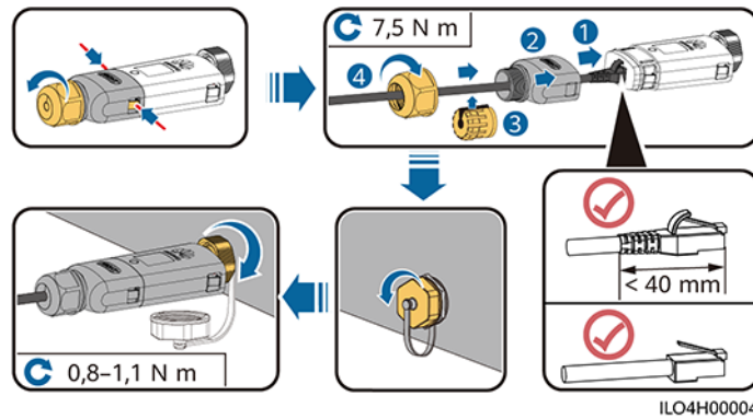
Figura 5-35 Instalación de un Smart Dongle WLAN-FE (comunicación FE)
