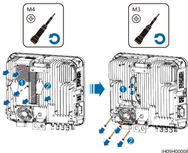
Figura 8-1 Desinstalación del ventilador defectuoso (Tipo 1)
