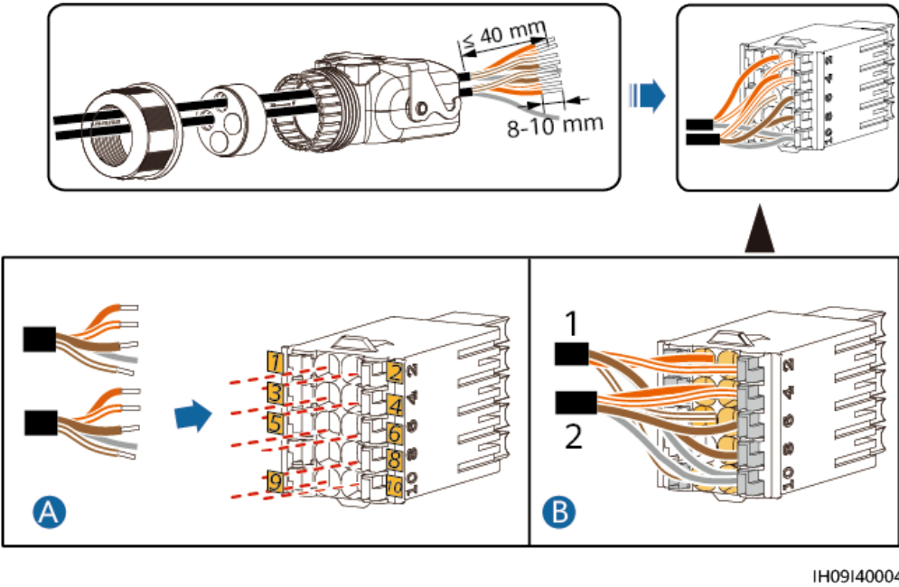
Figura 5-27 Instalación de los cables
