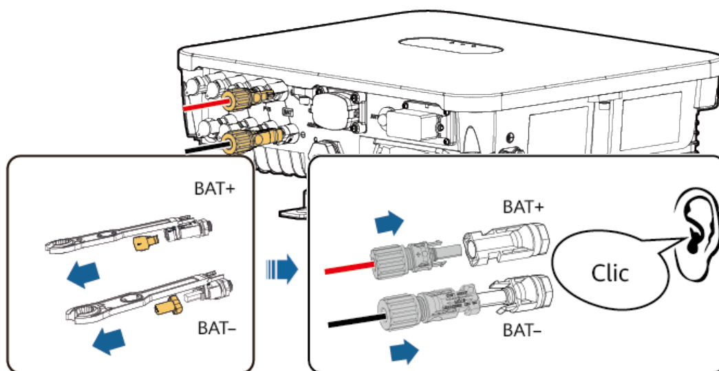
Figura 5-12 Conexión de los cables de las baterías
