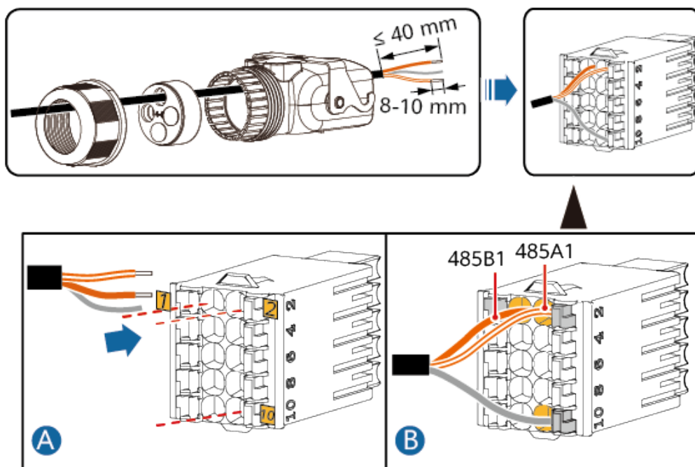
Figura 5-19 Instalación del cable
