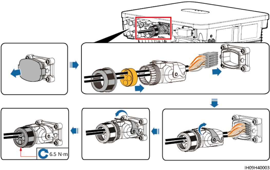
Figura 5-28 Fijación del conector del cable de señal
