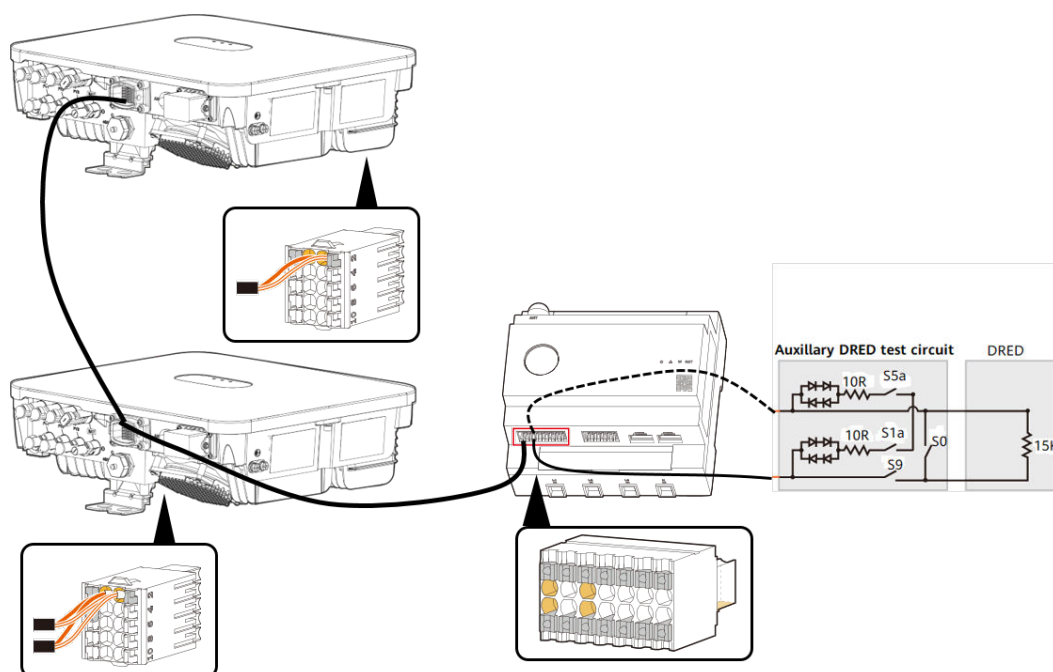
Figura 7-10 Diagrama de cableado para la función de DRM
