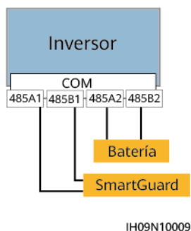
Figura 5-16 Conexión a red del SmartGuard (los componentes opcionales están encerrados en recuadros de rayas pequeñas)
