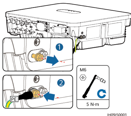
Figura 5-3 Conexión del cable de tierra
