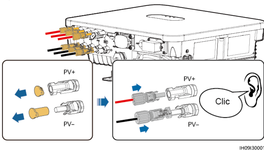
Figura 5-10 Conexión de los cables de entrada de CC
