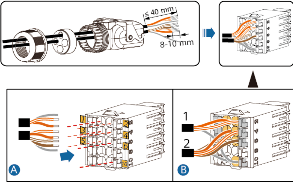
Figura 5-23 Instalación de los cables (conexión al EMMA y a la batería)
