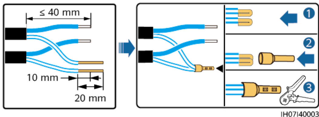
Figura 5-17 Engaste de dos cables de señal
