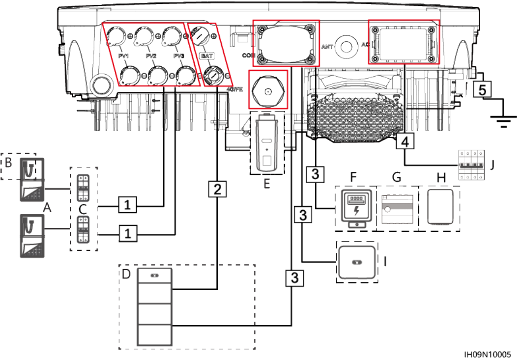
Figura 5-1 Conexiones de los cables del SUN2000 (los componentes encerrados en cuadros de rayas pequeñas son opcionales)
