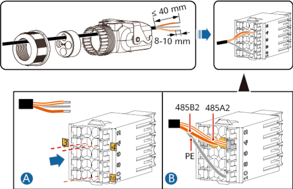
Figura 5-30 Instalación del cable (conexión al contador de potencia)
