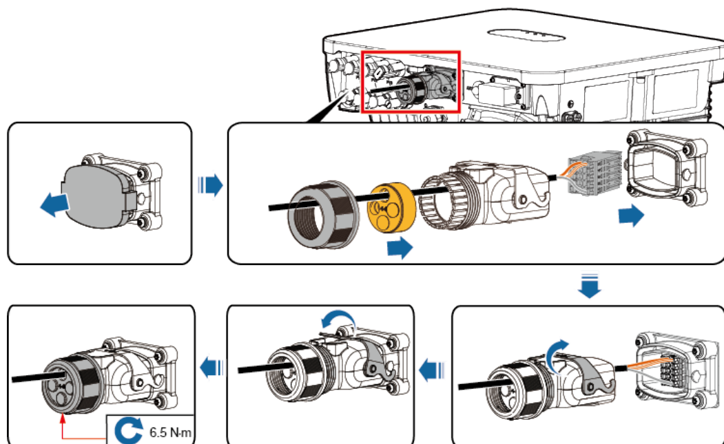
Figura 5-20 Fijación del conector del cable de señal
