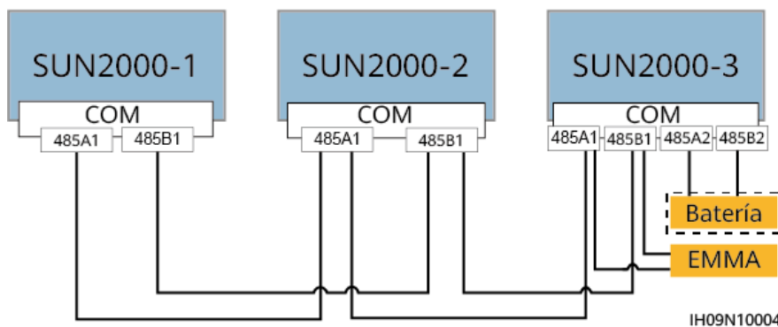
Figura 5-15 Conexión a red del EMMA (el componente encerrado en el cuadro de rayas pequeñas es opcional)
