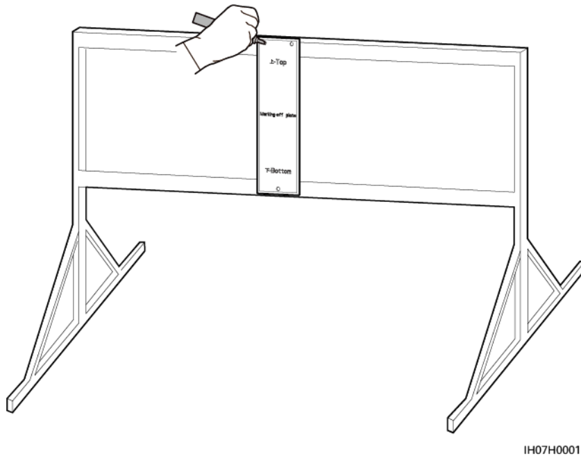
Figura 4-11 Determinación de las posiciones de los orificios
