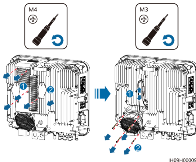
Figura 8-2 Desinstalación del ventilador defectuoso (Tipo 2)
