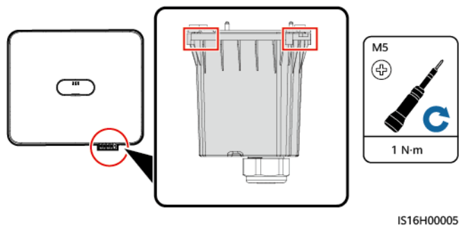
Figura 4-10 Instalación de una caja de derivación
