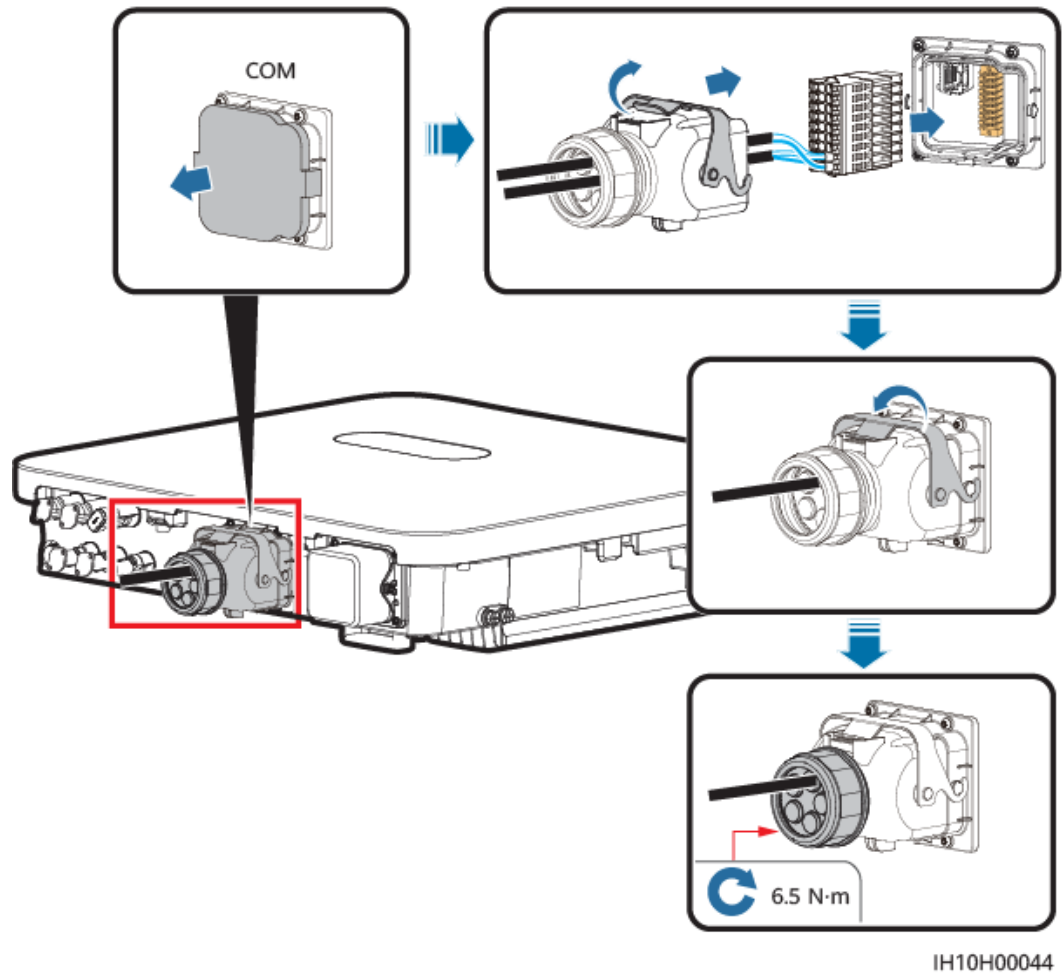
Figura 5-40 Fijación del conector del cable de señal
