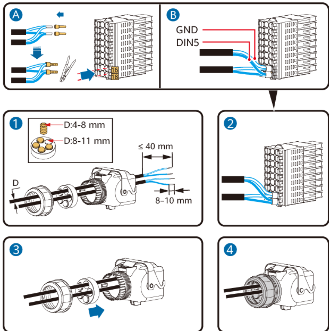
Figura 5-33 Instalación del cable
