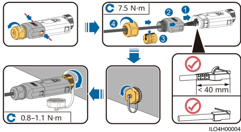
Figura 5-43 Instalación de un Smart Dongle WLAN-FE (comunicación FE)
