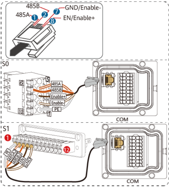
Figura 5-41 Conexión de los cables
