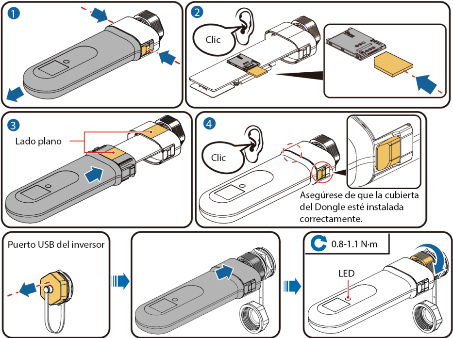
Figura 5-45 Instalación del 4G Smart Dongle (SDongleB-06)
