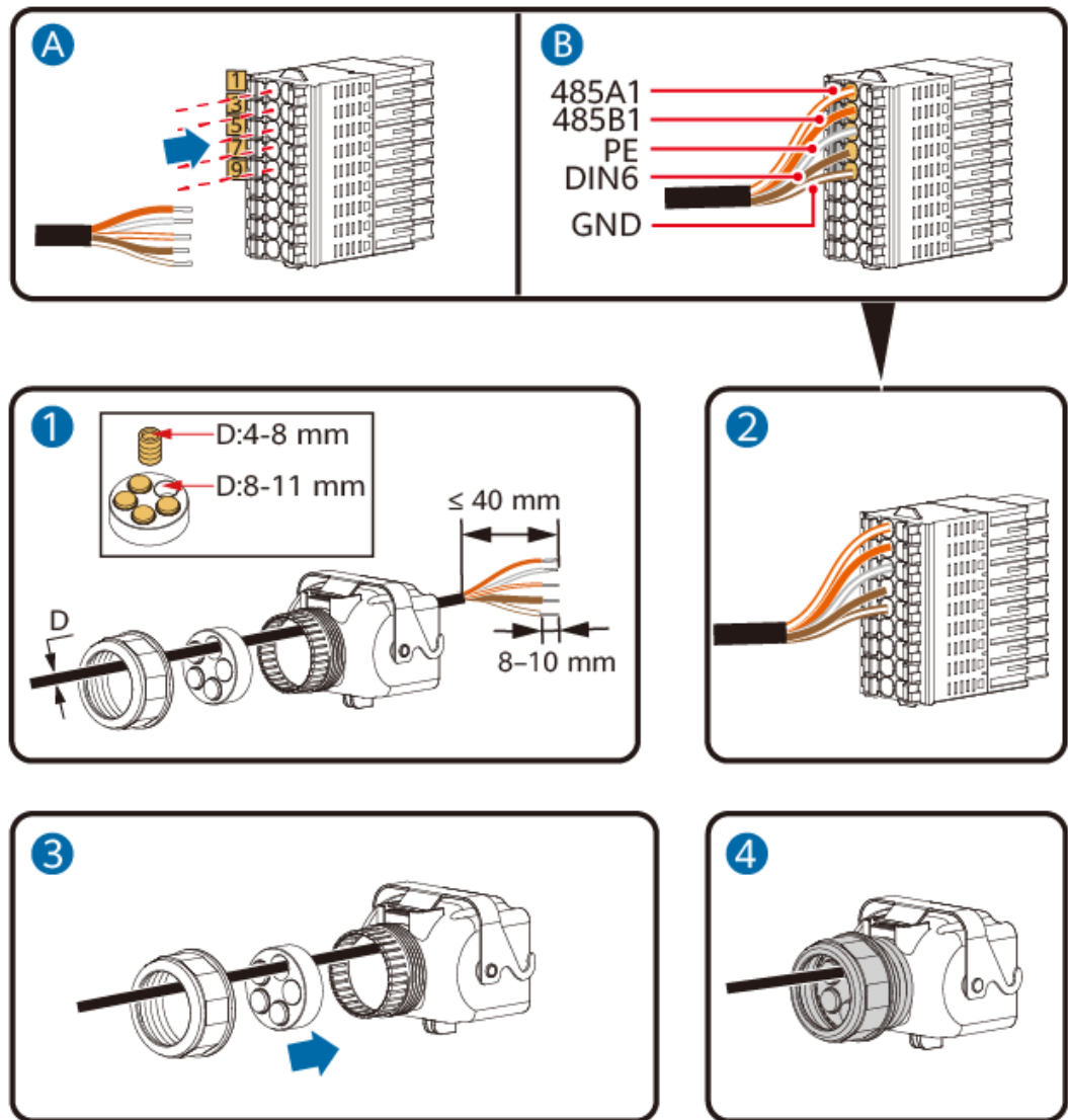
Figura 5-30 Instalación del cable
