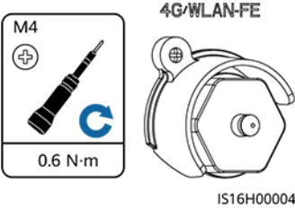
Figura 5-46 Instalación de componentes antirrobo para el Smart Dongle
